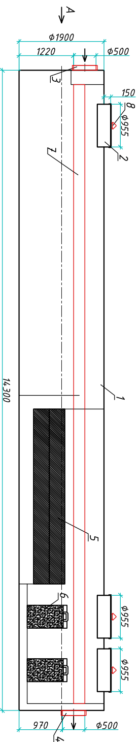
Разрез 1-1
